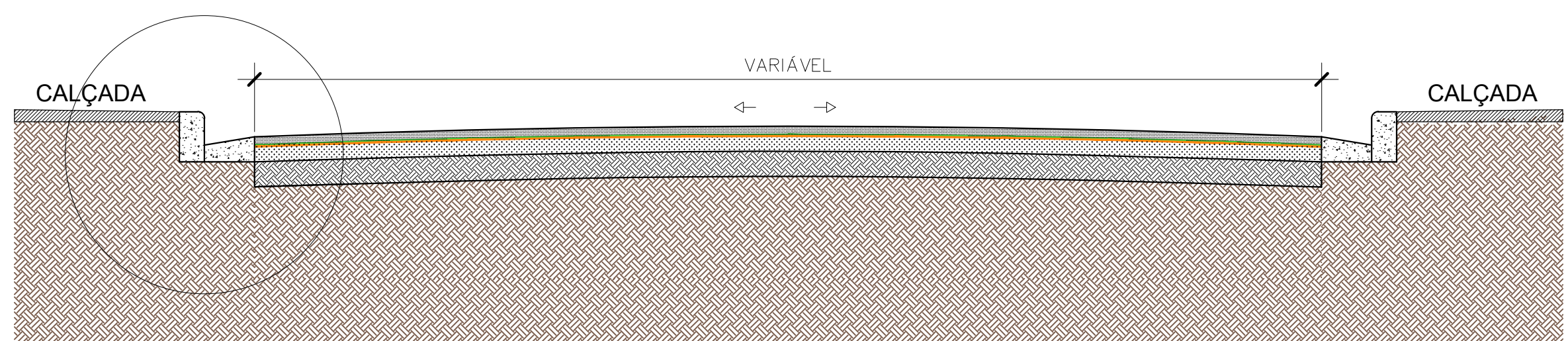
PERFIL TRANSVERSAL Escala 1/30
