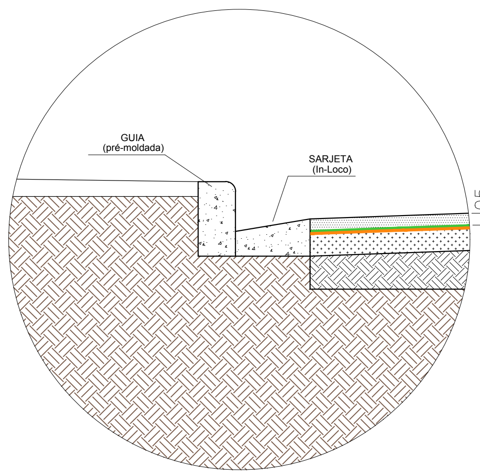
DETALHE Escala 1/15
