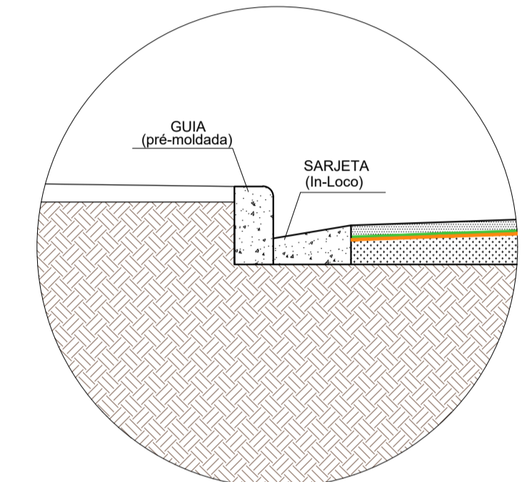
DETALHE 1 Escala: 1/20
