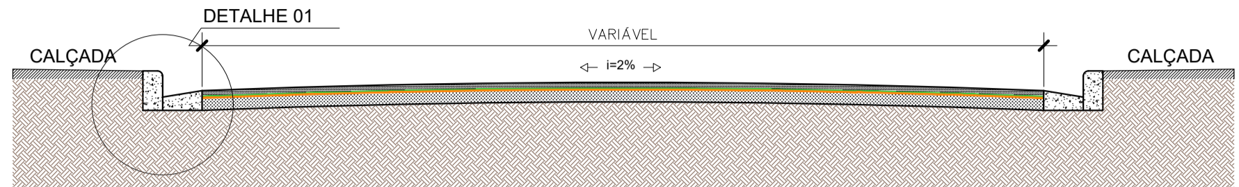
PERFIL TRANSVERSAL TÍPICO - RECAPE Escala: 1/40
