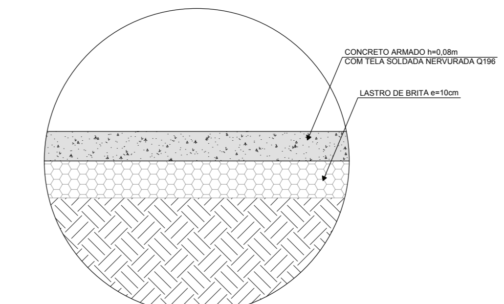
DETALHE PAVIMENTO DE CONCRETO (CALÇADAS) Escala 1/10
