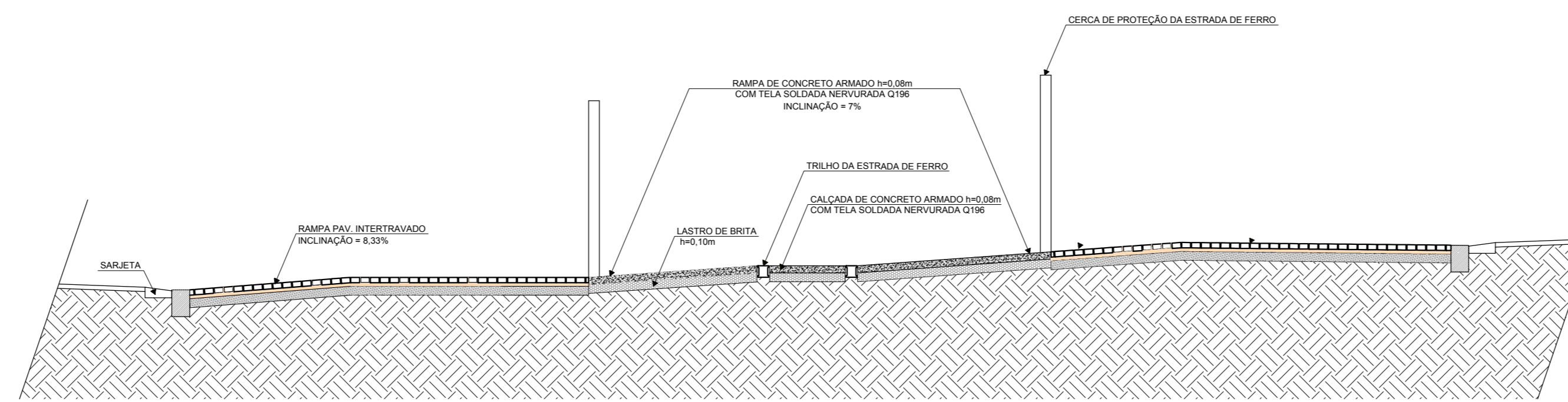
DETALHE CALÇADA DA TRAVESSIA DE PEDESTRES PELA ESTRADA DE FERRO Escala 1/50
