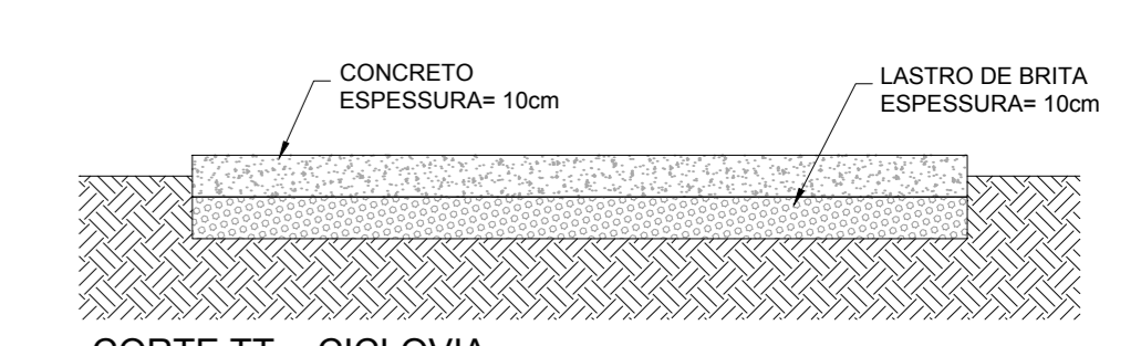
CORTE TT - CICLOVIA
