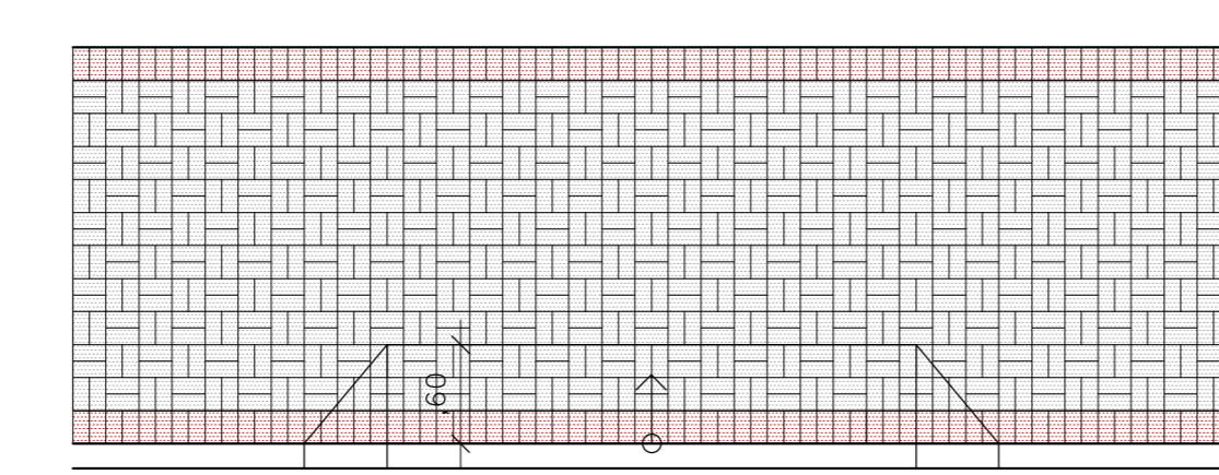
DETALHE RAMPA PARA ACESSO DE VEÍCULOS Escala 1/50
