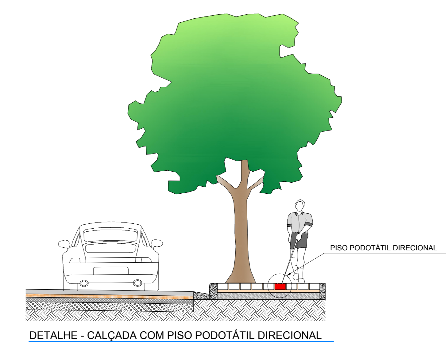
DETALHE - CALÇADA COM PISO PODOTÁTIL DIRECIONAL ESCALA 1/15
