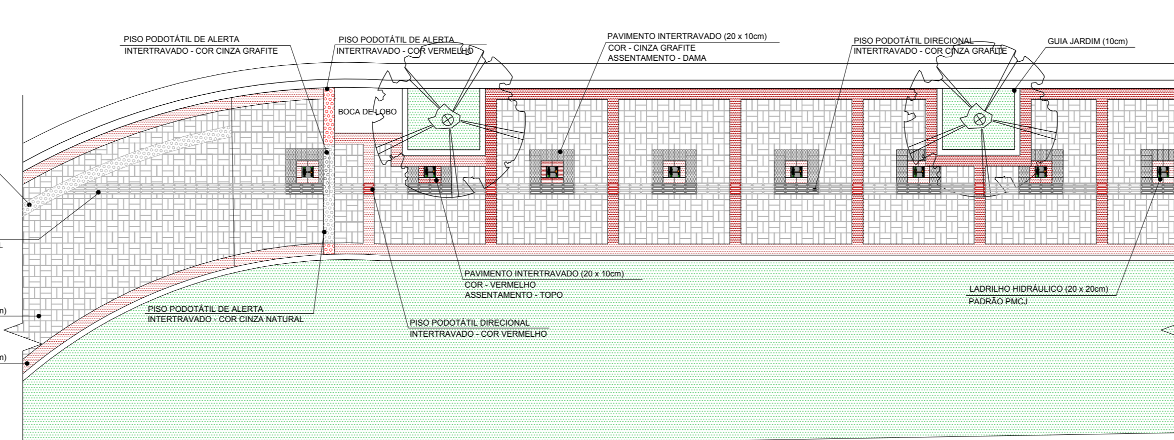
DETALHE TÍPICO DE CALÇADA EM INTERTRAVADO SEM ESCALA
