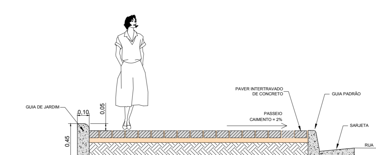
PERFIL TRANSVERSAL - CALÇADA PAV. INTERTRAVADO Escala 1/20
