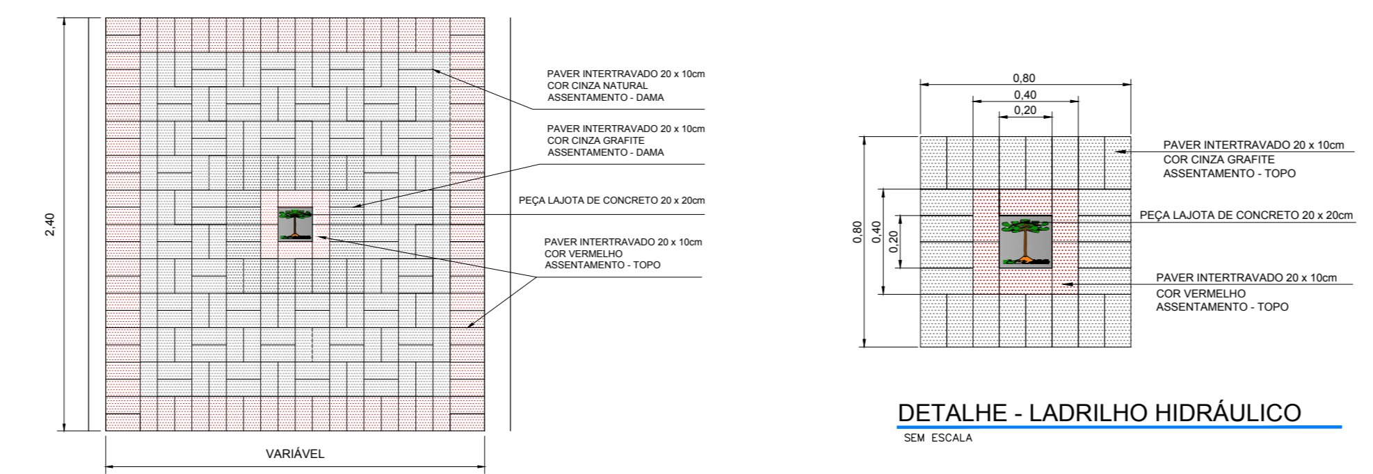
DETALHE - PAGINAÇÃO CALÇADA EM PAVIMENTO INTERTRAVADO SEM ESCALA
