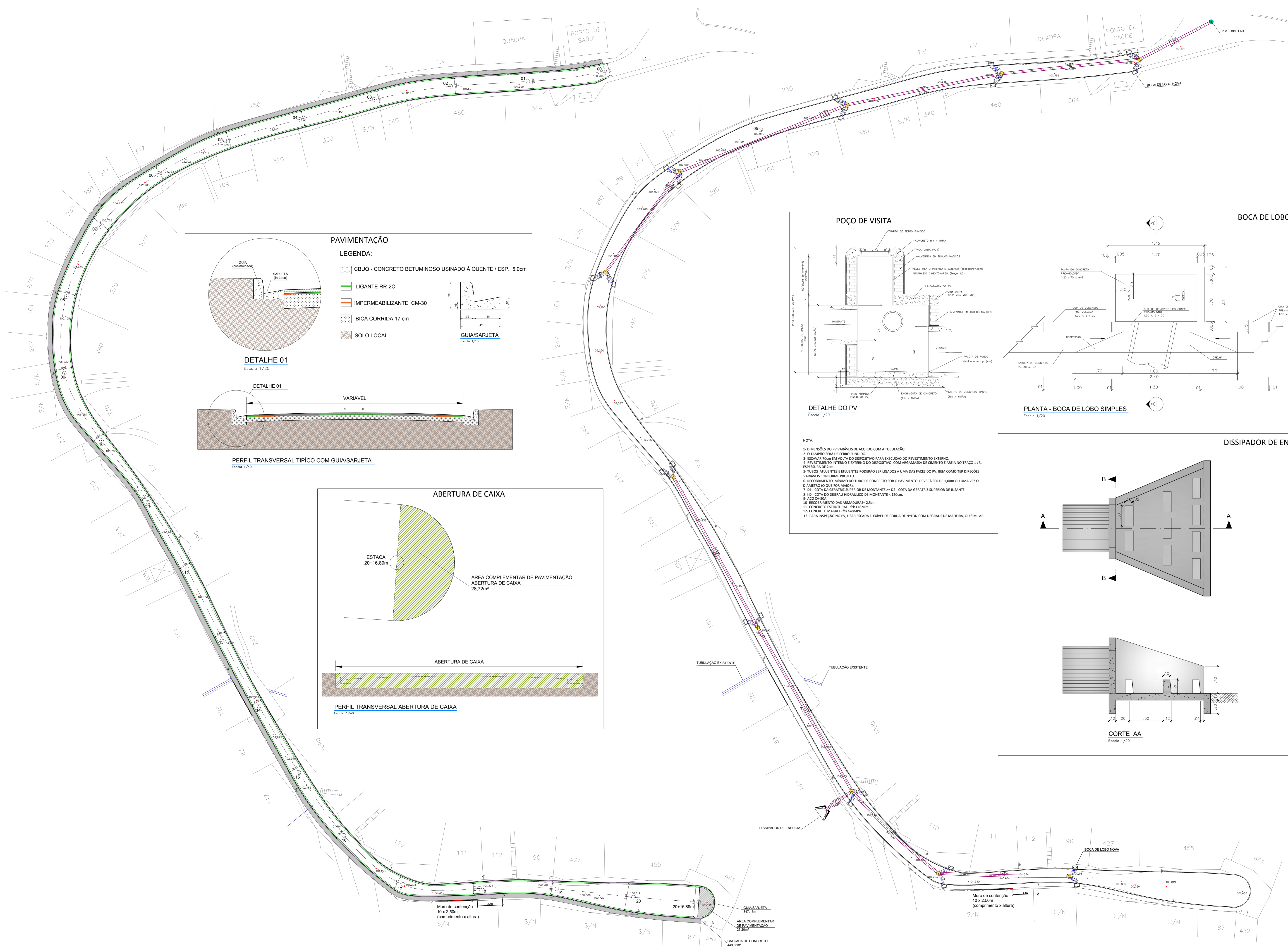
PLANTA DE DRENAGEM Escala 1/350 MEDIDAS EM METROS
