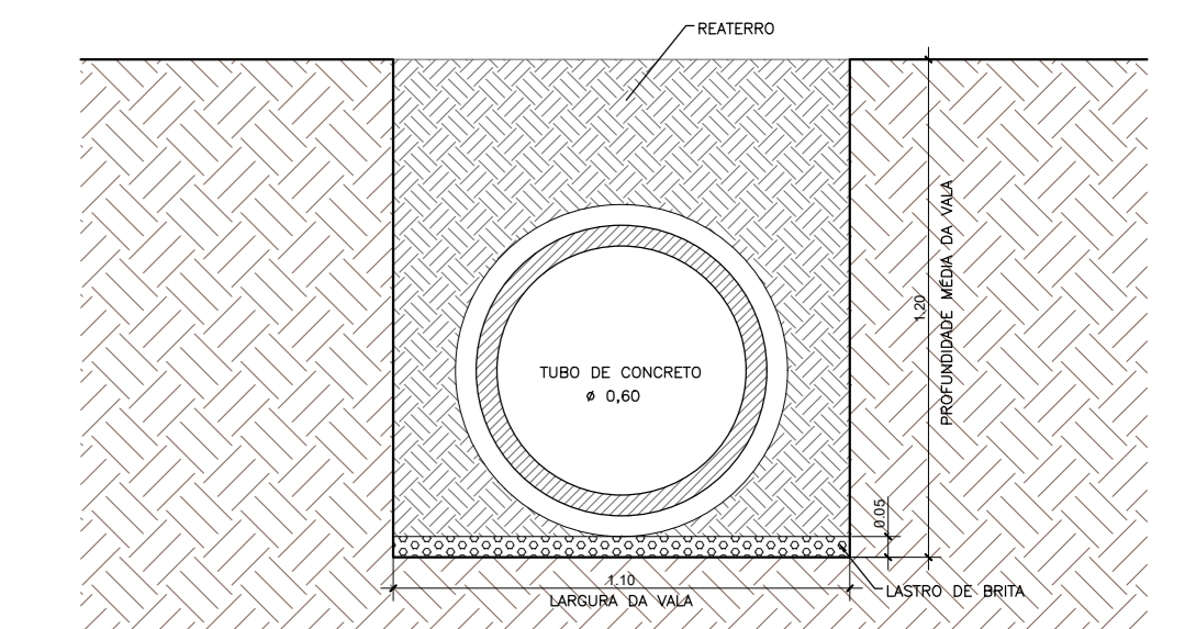
SEÇÃO TRANSVERSAL - VALA DE ASSENTAMENTO DOS TUBOS 600mm
