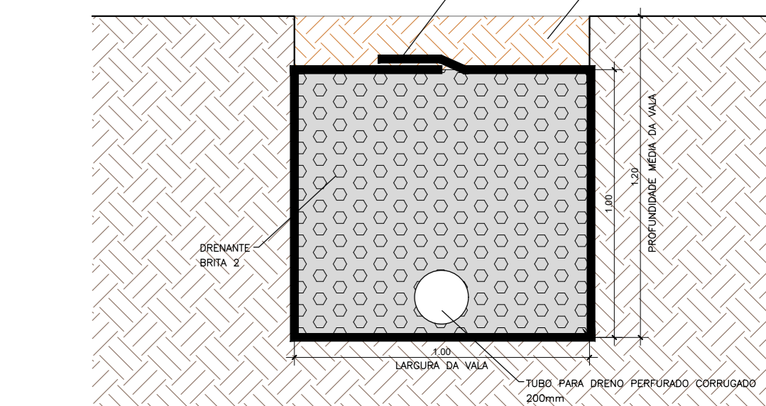
SEÇÃO TRANSVERSAL - DRENO
