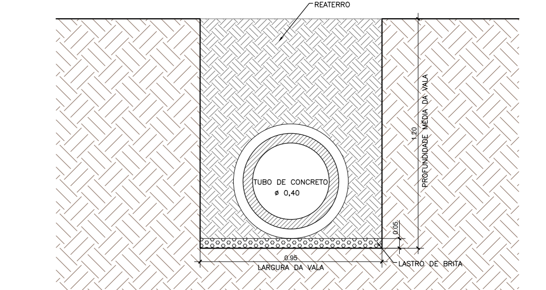
SEÇÃO TRANSVERSAL - VALA DE ASSENTAMENTO DOS TUBOS 400mm
