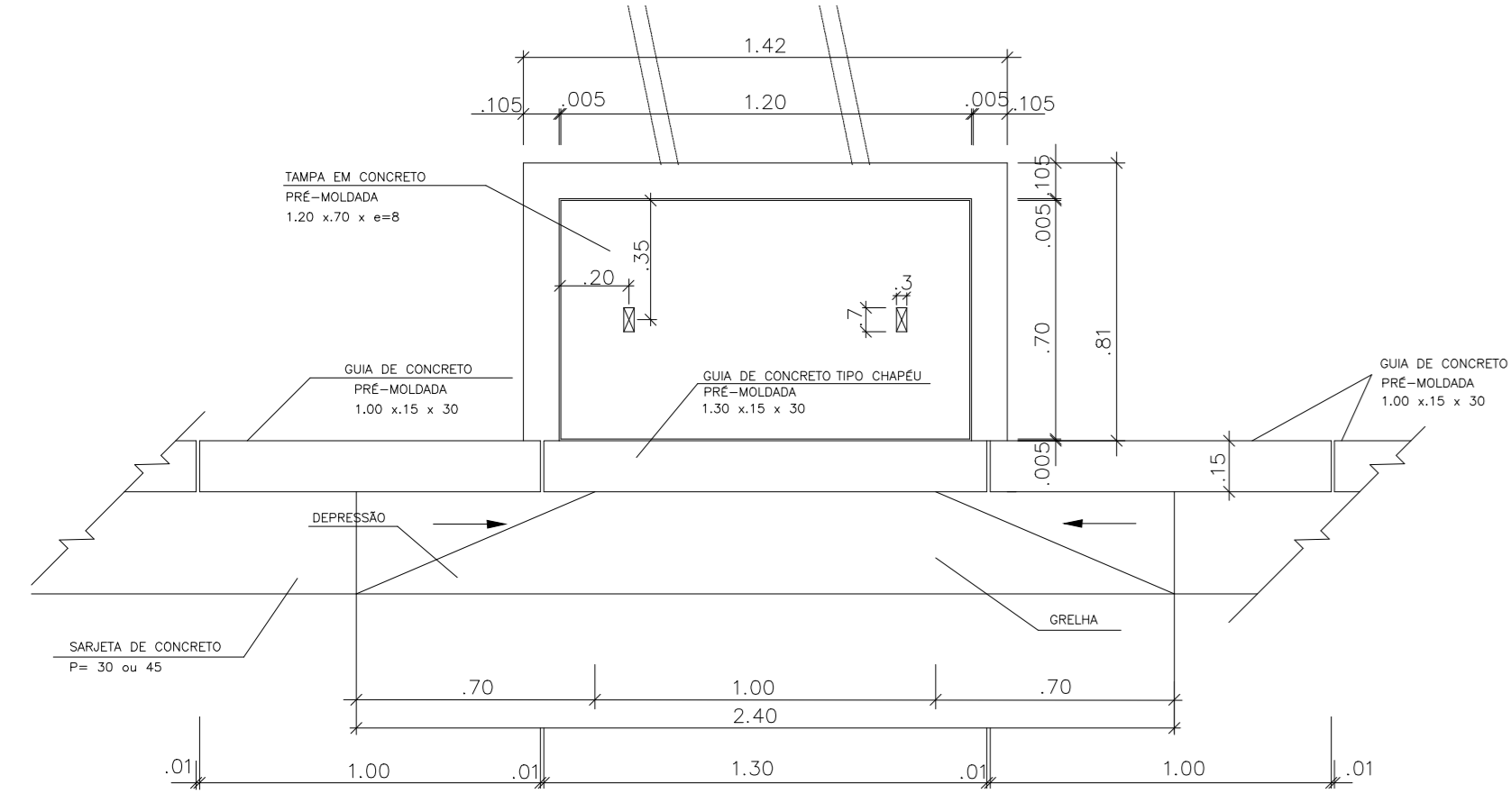
PLANTA - BOCA DE LOBO SIMPLES
