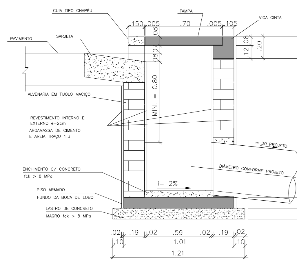
CORTE - BOCA DE LOBO
