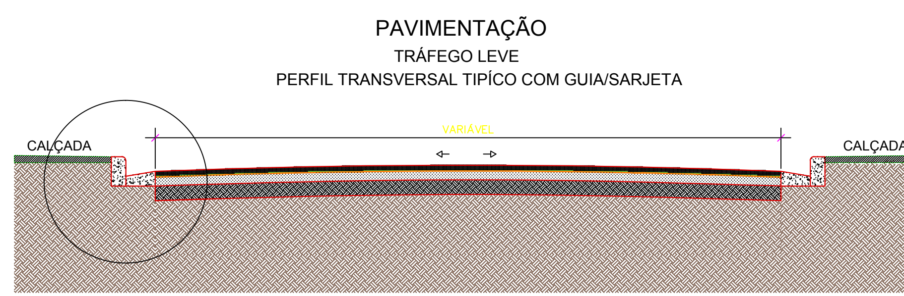
PERFIL TRANSVERSAL Escala: 1/40
