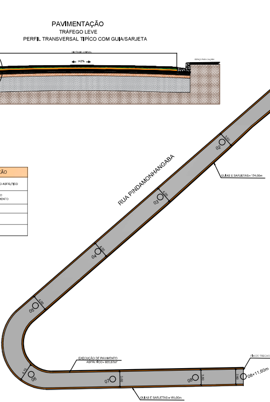
PLANTA DE EXECUÇÃO Escala 1/200
