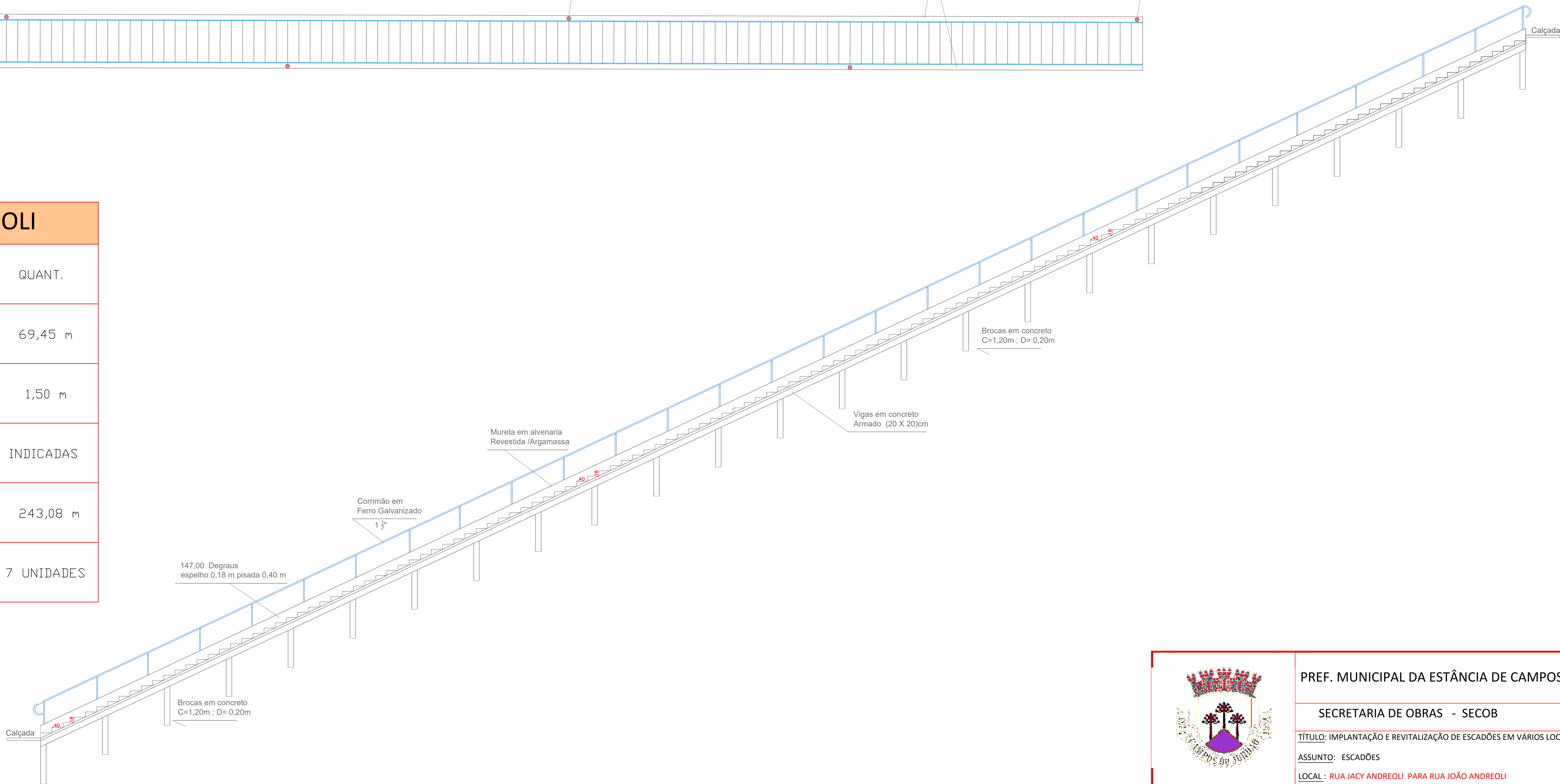
PERFIL LONGITUDINAL Esc: 1:100
