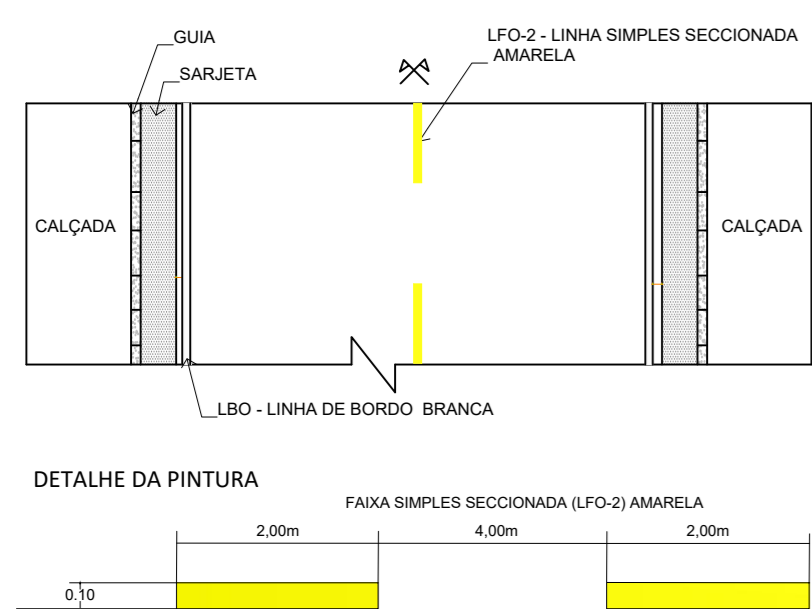
RUA MONTE NEGRO ESC: 1:250
