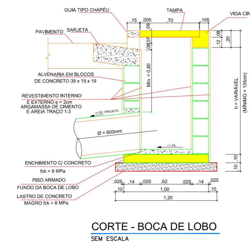
CORTE - BOCA DE LOBO SEM ESCALA
