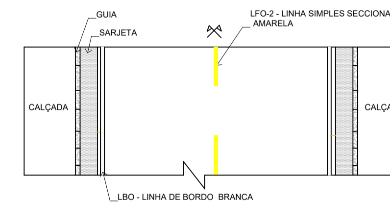
DETALHE DA PINTURA
