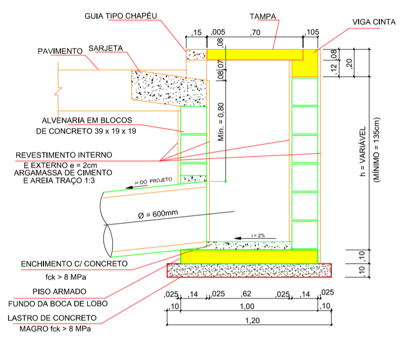
CORTE - BOCA DE LOBO SEM ESCALA
