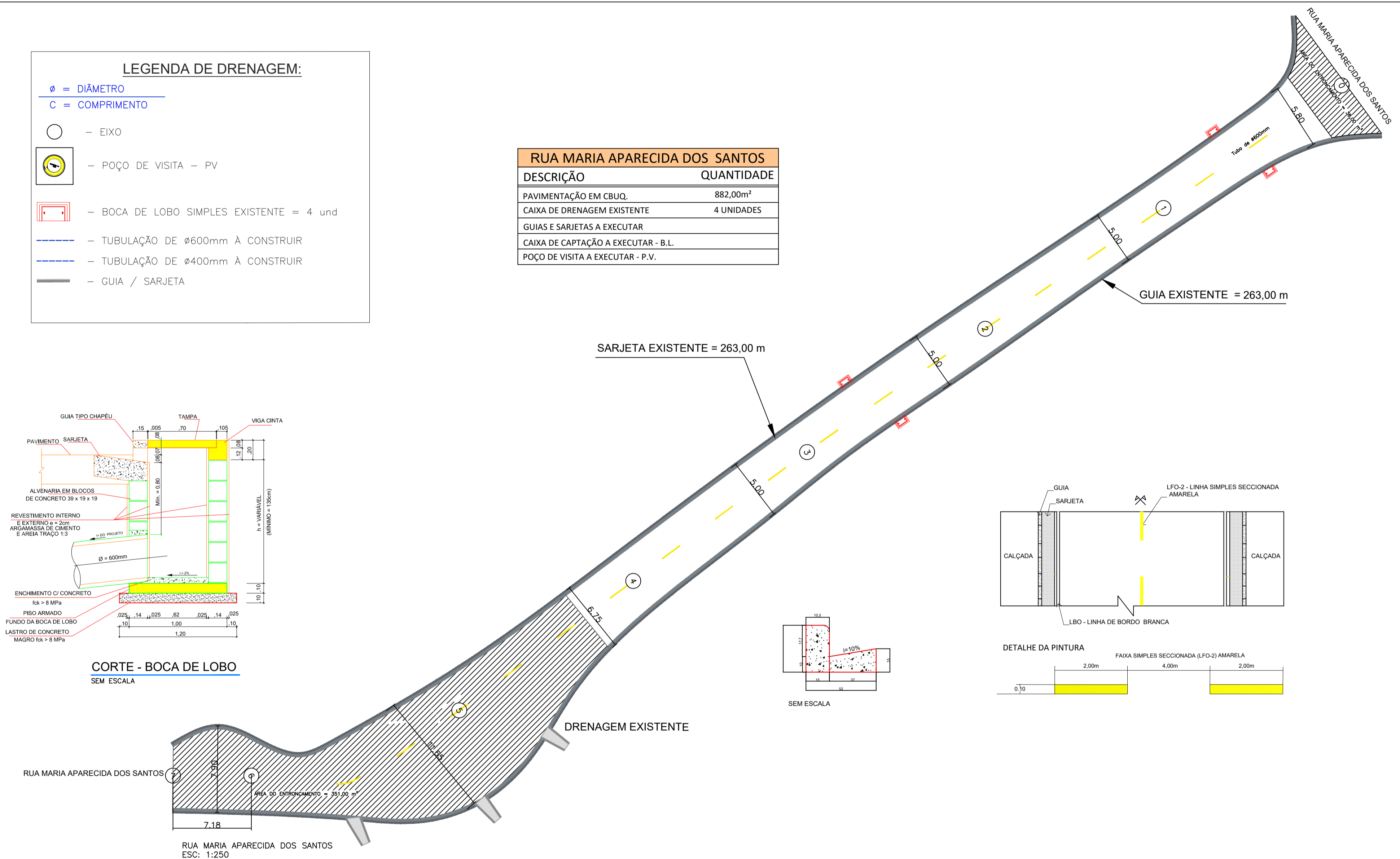
DETALHE DA RUA
