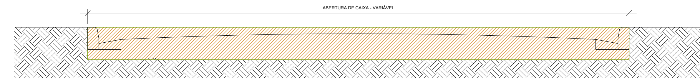
SEÇÃO - ABERTURA DE CAIXA PARA PAVIMENTO ASFÁLTICO (CUBUQ) Escala 1/50
