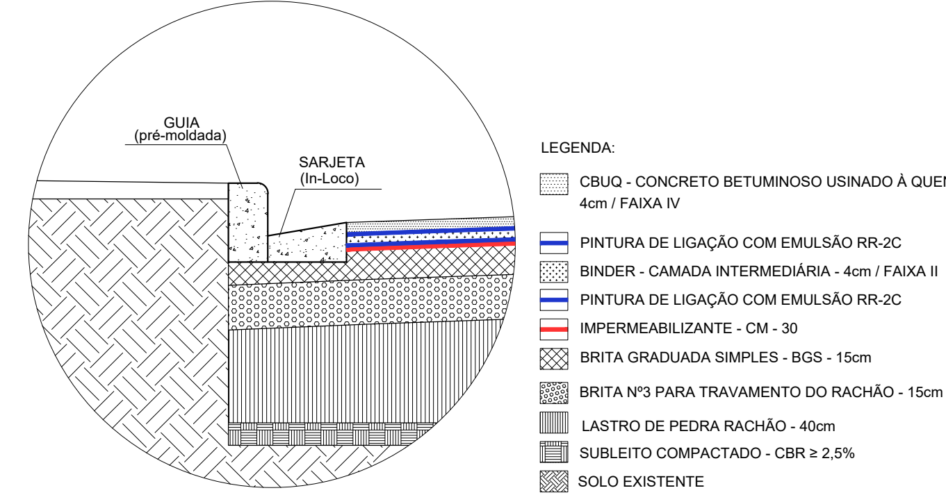
DETALHE 01- PAVIMENTAÇÃO COM REFORÇO DE BASE
