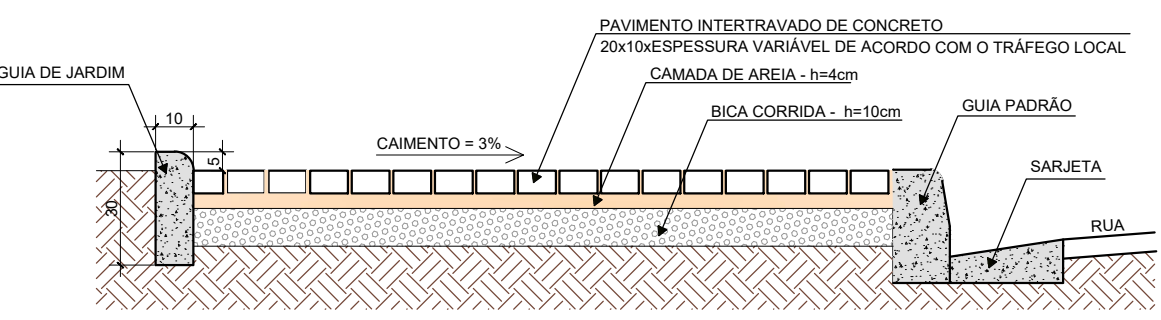
SEÇÃO TRANSVERSAL - CALÇADA EM PAVIMENTO INTERTRAVADO Escala 1/20
