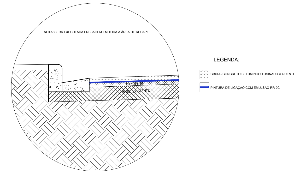
DETALHE RECAPEAMENTO
