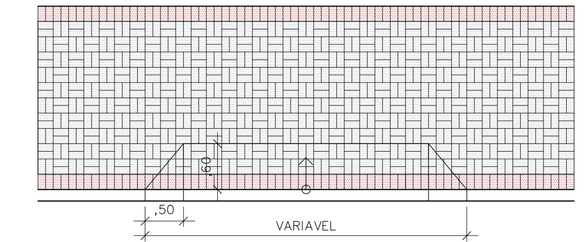
DETALHE RAMPA PARA ACESSO DE VEÍCULOS Escala 1/50
