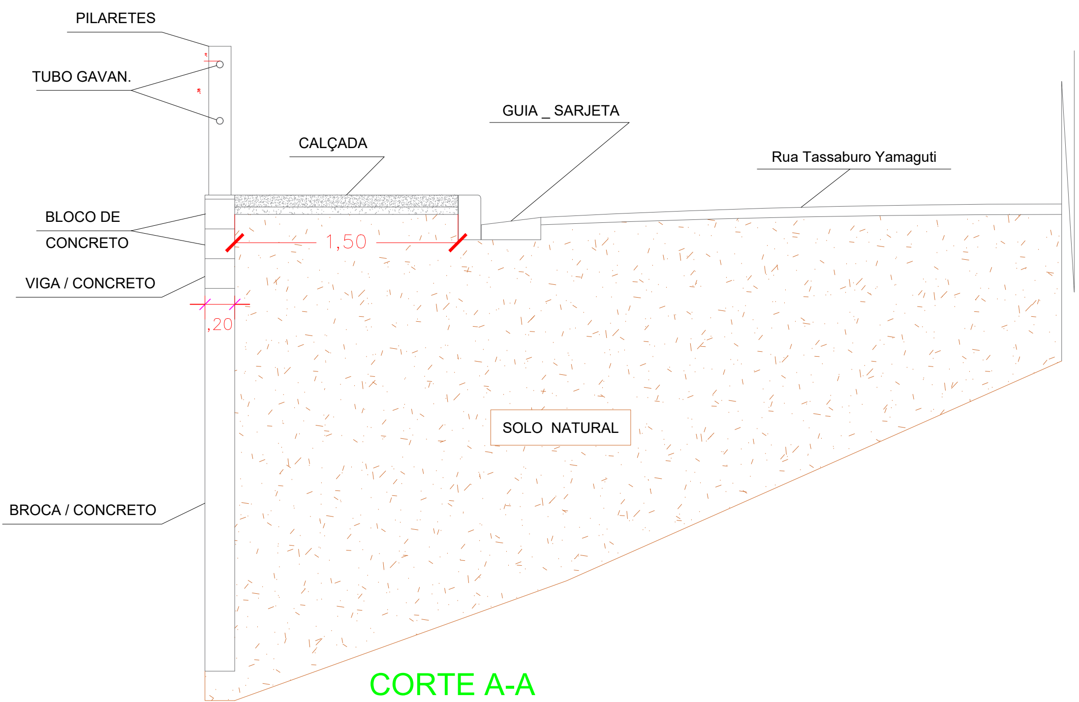
CORTE A-A
